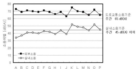
[그림 1] 공동주택 외벽 도달 도로소음 및 실내소음 측정결과
