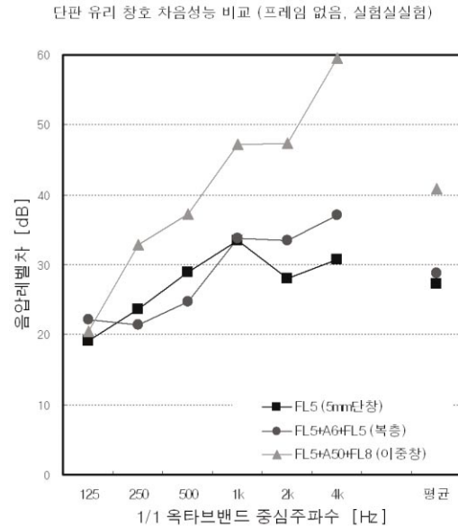
[그림 7] 단일유리의 차음성능 (실험실)
