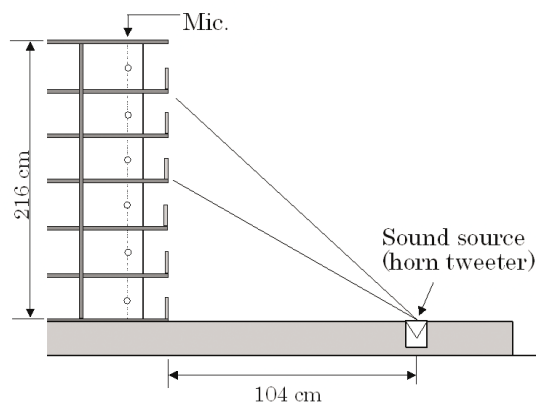
[그림 13] 도로교통소음의 전달 모형실험
