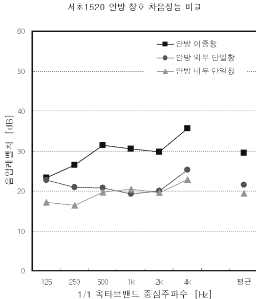
[그림 8] 창호의 차음성능 (현장)
