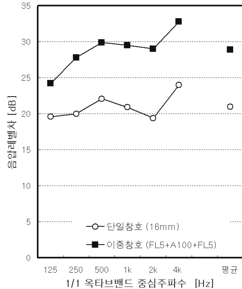
[그림 9] 주거성능실험동에서의 창호 차음성능 측정결과
